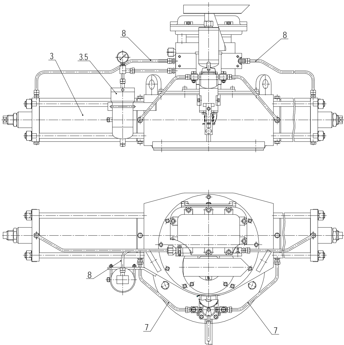
Рисунок А.6 – Пневмогидропривод
