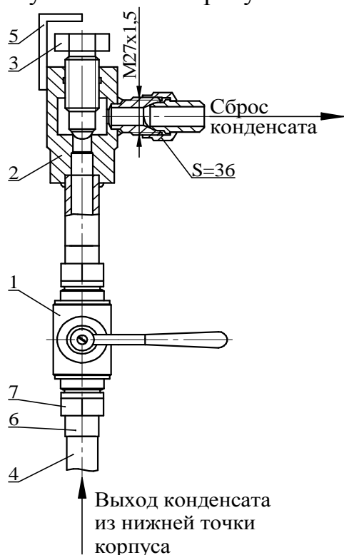
Рисунок 6 – Узел дренажный
