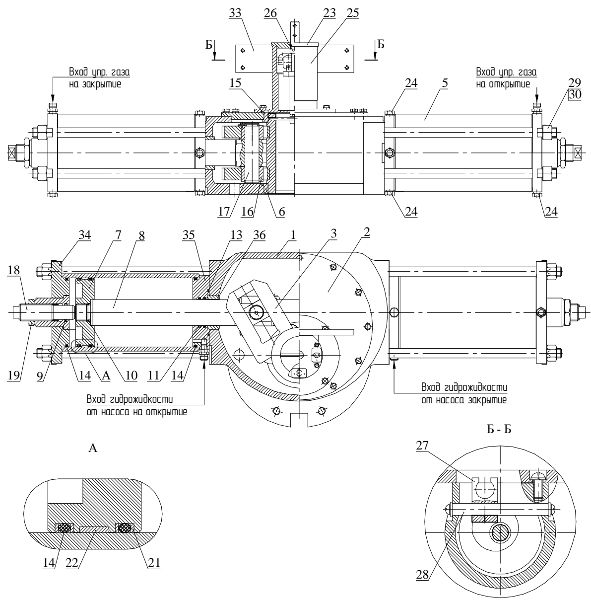
Рисунок А.7 – Привод
