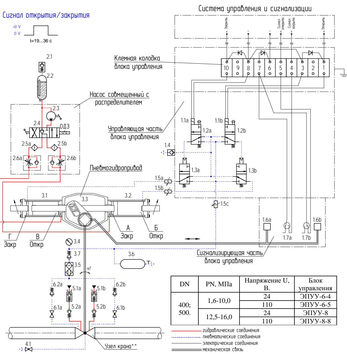
Рисунок А.11 – Схема управления с ЭПУУ-6 и ЭПУУ-8 с разделенными цепями управления и сигнализации (шестипроводная)
