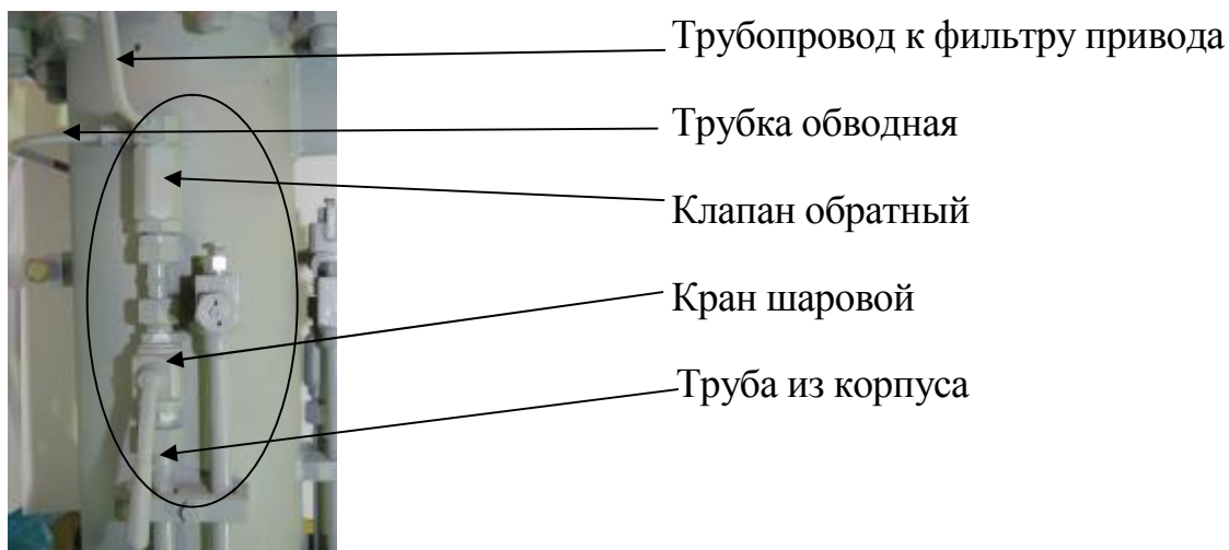
Рисунок 8 – Трубопровод управляющего газа
