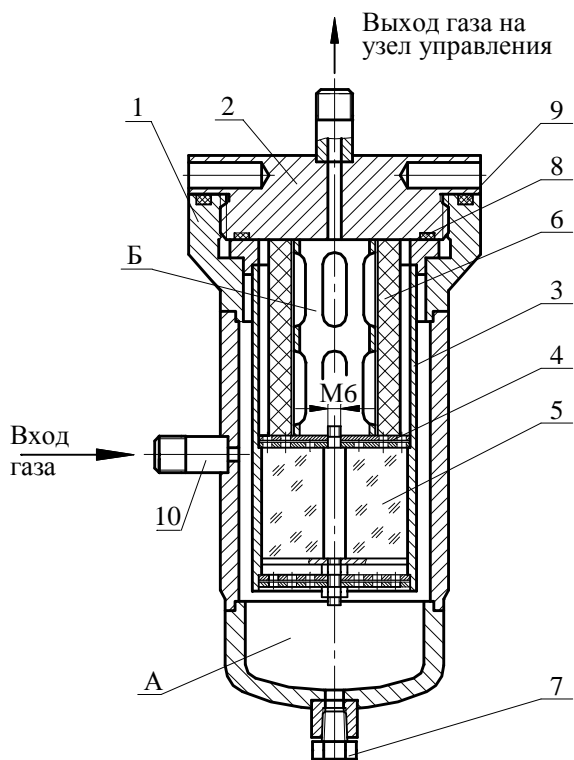
Рисунок 11 – Фильтр-осушитель газа
