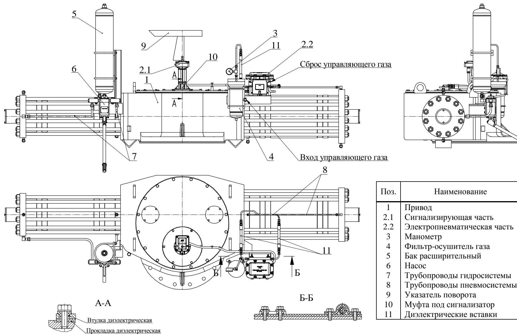
Рисунок А.6 – Пневмогидропривод
