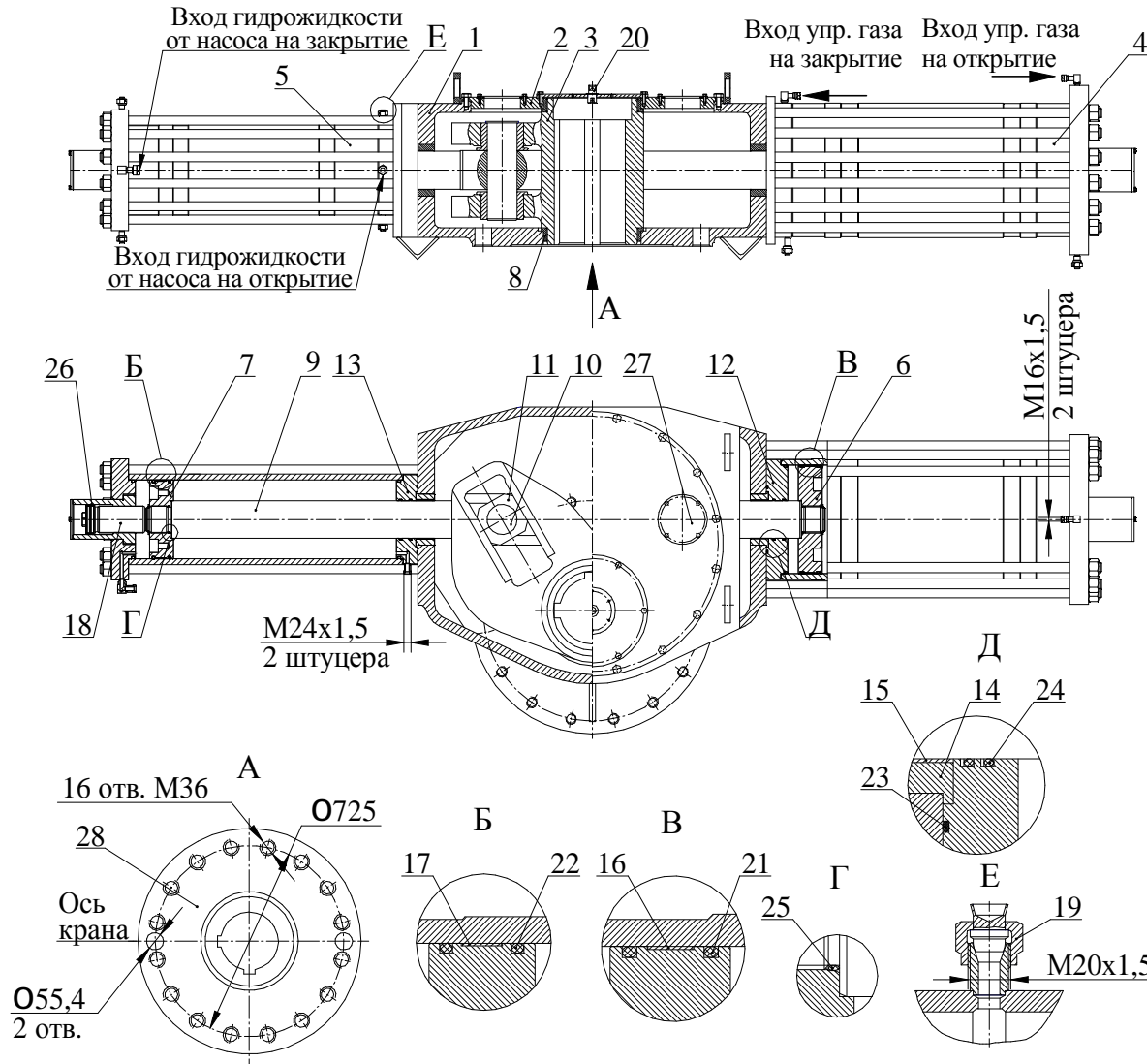
Рисунок А.7 –Привод
